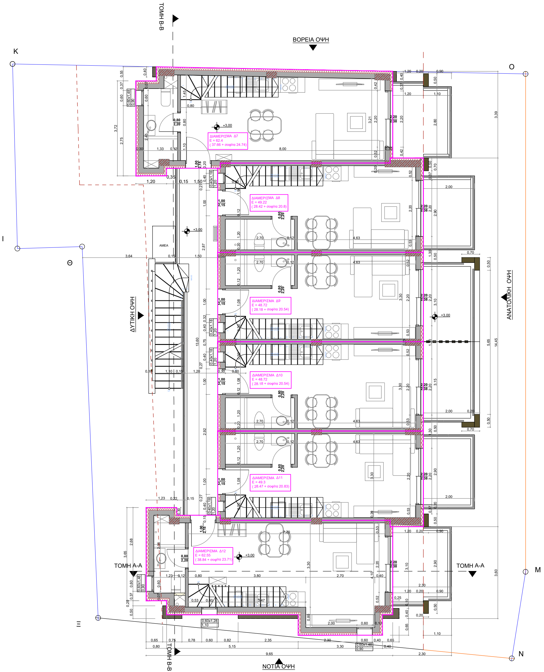
ΚΑΤΩΦΗ 1 ου ΟΡΟΦΟΥ
